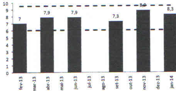
Figura 3 - pH
