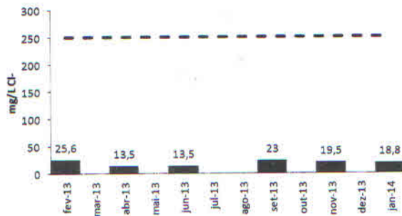
Figura 5 - Cloreto (mg/L)
